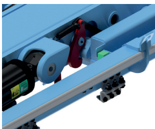
1. Verrouillage médian mécanique. Permet le transport de caisses de différentes longueurs.
