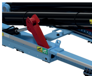
2. Démultiplicateur de force à l'inclinaison breveté, conçu pour augmenter la force de levage au démarrage, avec rouleaux permettant le mouvement horizontal sans frottement.
